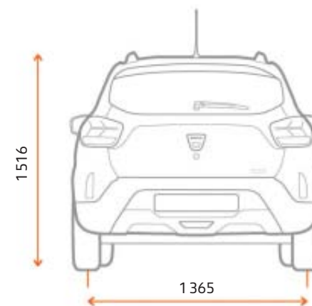
VUE ARRIÈRE
